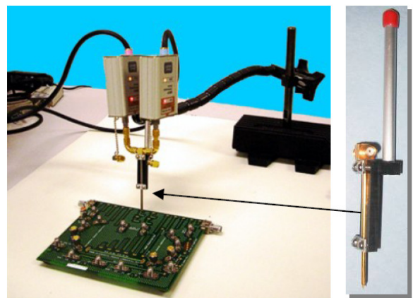
그림 2) Tektronix의 PPM100 Articulating Arm에 직접 연결한 모습- 기본 구성품인 GPMMA 어댑터를 이용해 보다 고대역의 정밀한 TDR 측정. 제조사에 상관없이 거의 모든 종류의 Probe Manipulator에 연결 가능
