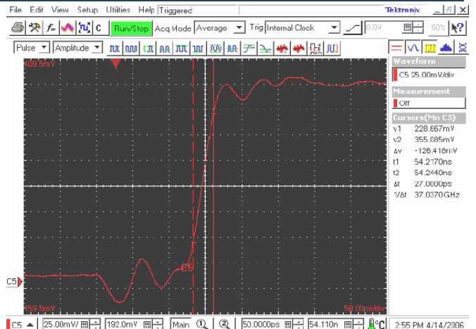
그림 6) Differential Rise Time – 9ps TDR pulser 출력을 DSA8200과 50GHz module로 측정된 Gigaprobe의 Rise Time. 대역폭이 30GHz를 상회한다.
