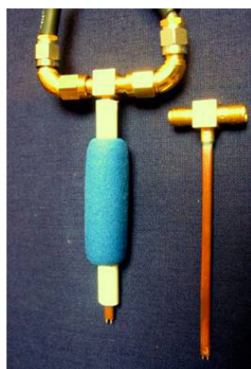
그림 1) 편리한 Hand Held 프로빙- EZ-hold 쿠션 어댑터를 사용해 미세한 간격의 포인트에 쉽게 프로빙할 수 있다.
