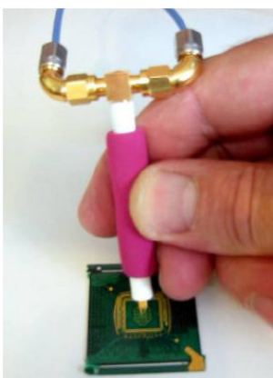
그림 1) 편리한 Hand Held 프로빙- EZ-hold 쿠션 어댑터를 사용해 미세한 간격의 포인트에 쉽게 프로빙할 수 있다.
