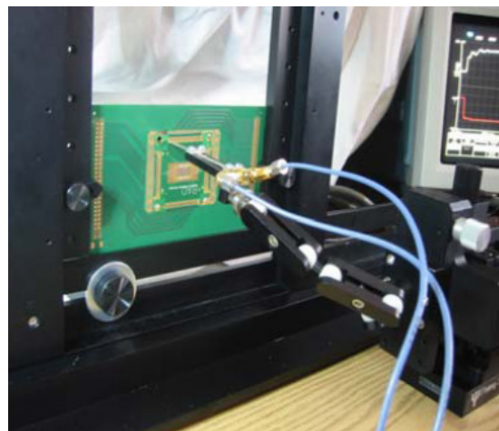
그림 8) 다양한 Probe Manipulator 로 수직 프로빙
