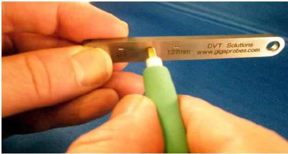
그림 3) Signal –Signal Pitch Calibration- Model 10 SMA Calibration 렌치로 빈번히 사용하는 0.8mm, 1.0mm, 1.27mm 간격을 조정. 프로빙 위치를 조정하고 이외의 다양한 간격을 정밀하게 조정하기 위해서는 기본 포함된 트위저와 탁상용 확대경을 사용.
